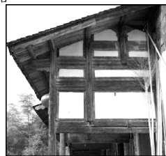
图7 举架露明的山墙形态
