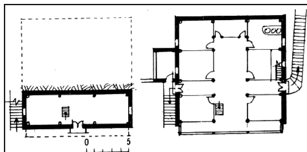
图3 兰汤村应宅平面(左为入口层,右为二层) [5]
