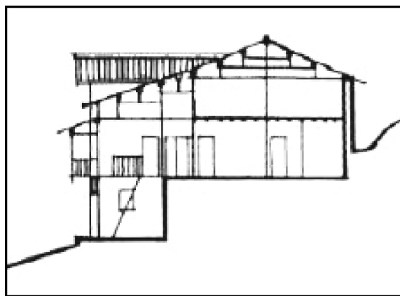
图4 兰汤村应宅剖面 [5]
