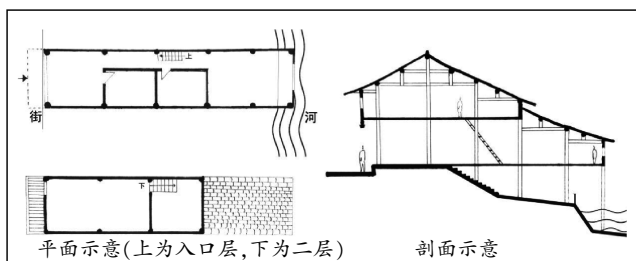
图5 武夷山南门街235号宅平面及剖面
