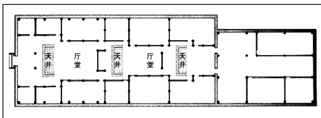
图1 下梅村儒学正堂平面 [3]
