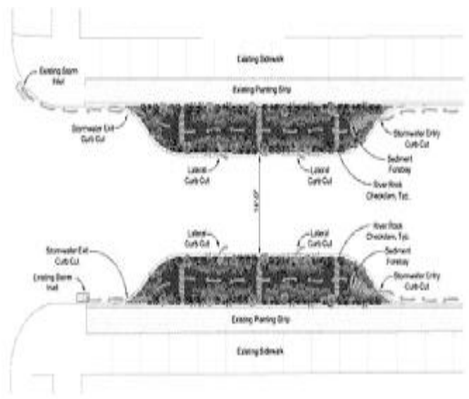
图9 水流示意图
