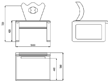
图 7 太极滑移座椅设计图
