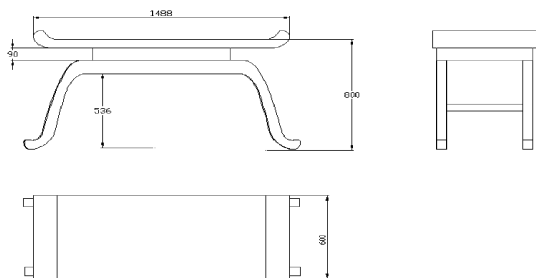
图 12 “天字形”书桌 CAD 总体尺寸设计图
