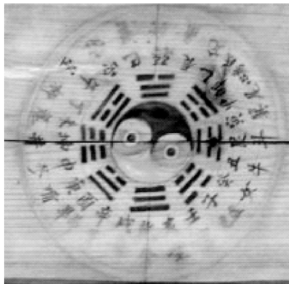
图 2 宝山太极图
