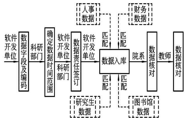
图2 高校信息化科研管理平台数据建设流程
